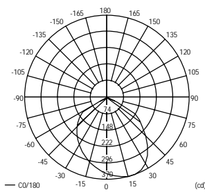
99 771 06-07: Photometrisches Diagramm mit Diffusor
